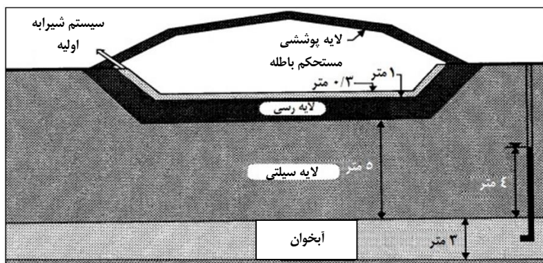
شکل ۲-۳- محصور کردن سطح انباشتگاه باطله با ایجاد یک لایه پوششی نفوذناپذیر
