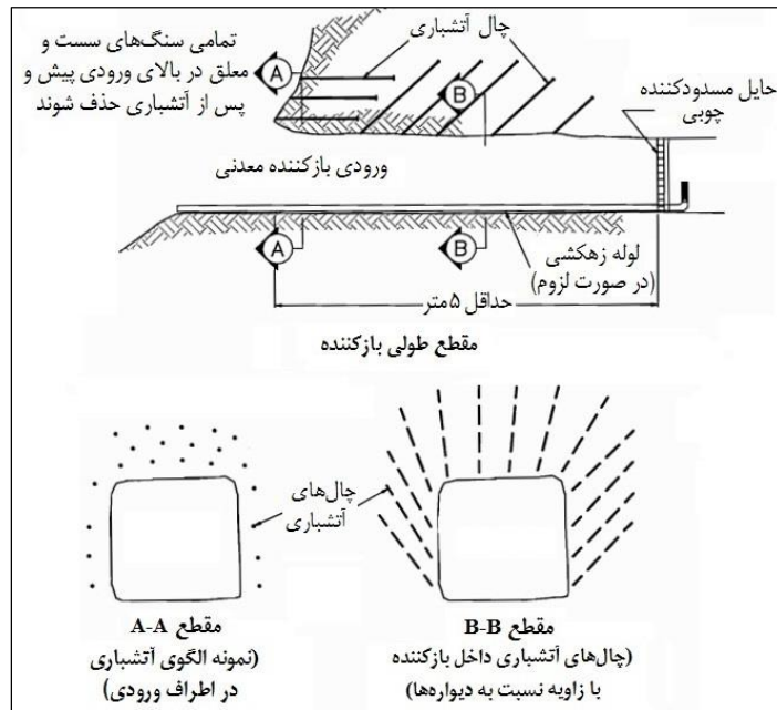
شکل ۲-۱۵- طرح کلی بستن بازکننده‌ها با آتشیاری
