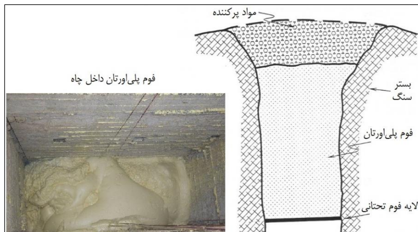
شکل ۲-۱۲ - نمونه‌ای از بستن چاه با مجرا بنده فوم پلی‌اورتان
