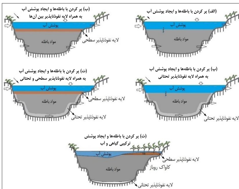
شکل ۳-۴- حالت‌های پر کردن کاواک با ترکیبی از مواد باطله و آب
