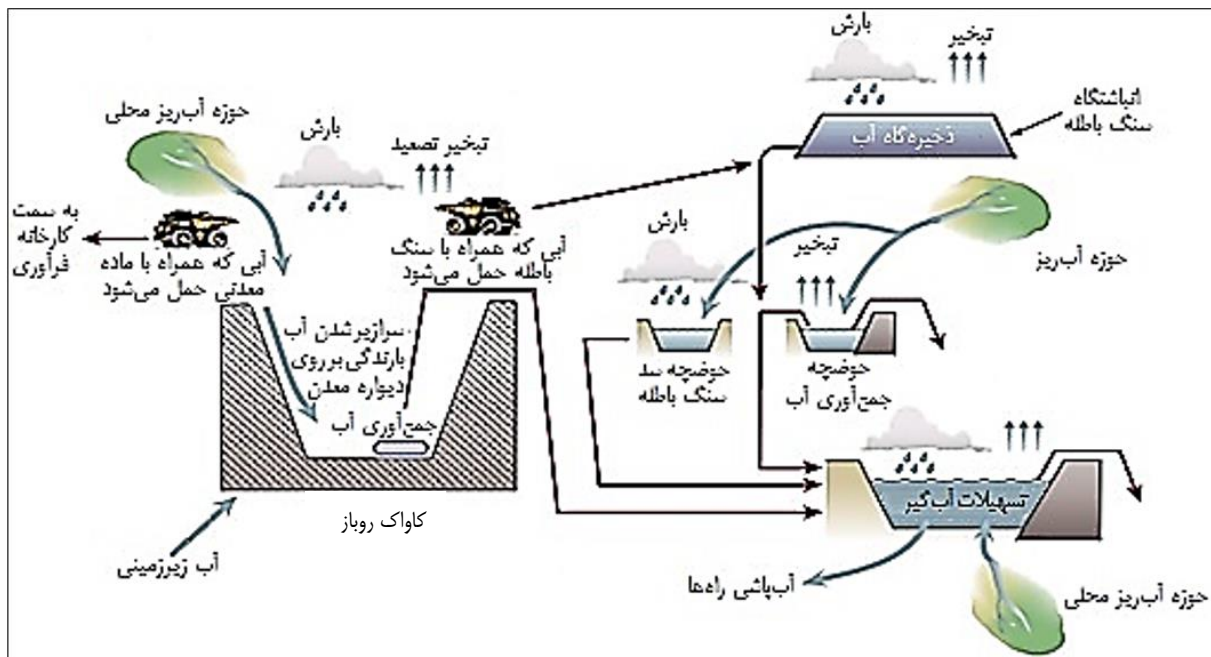
شکل ۲-۲- نحوه کنترل روانابها
