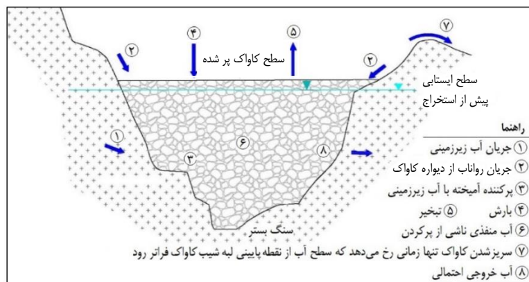
شکل ۳-۲- جزئیات پر کردن کاواک روباز با مواد باطله
