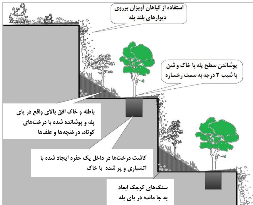
شکل ۳-۱- طرح مفهومی بازسازی معادن سنگ تزئینی و نما
