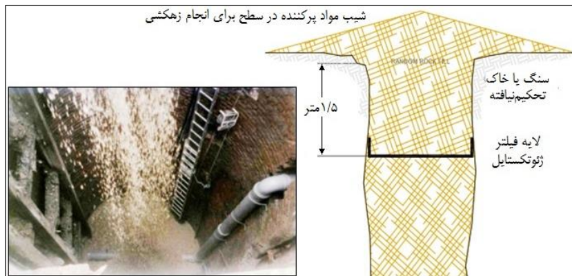
شکل ۲-۱۳- نمونه ای از بستن دائمی چاه با پر کردن
