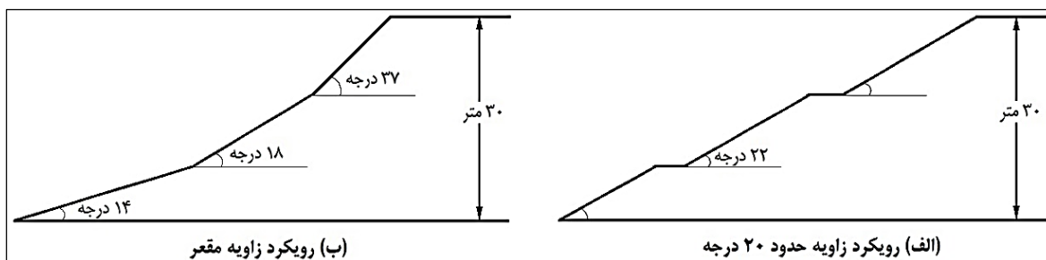
شکل ۲-۴- کاهش شیب نهایی دیواره انباشتگاه با شکستن آن به قطعه‌های با شیب کمتر: الف- شیب حدود ۲۰ درجه، ب- شیب مقعر
