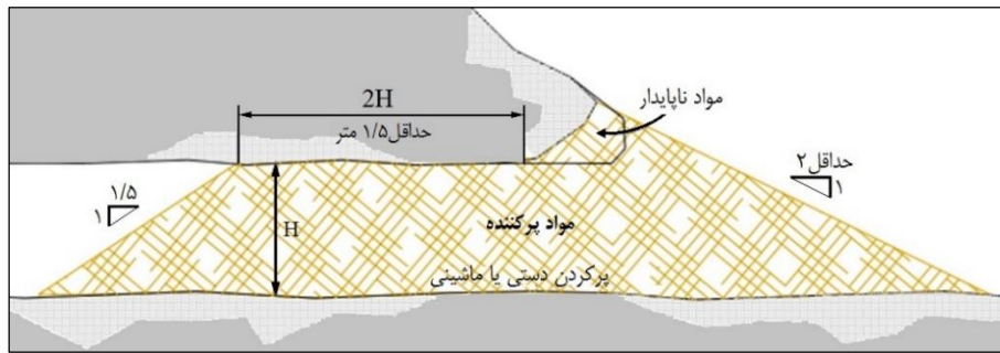
شکل ۲-۱۴- نمونه‌ای از بستن دایمی تونل با پر کردن
