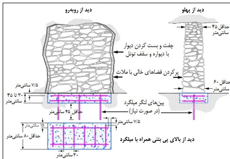
شکل ۲-۱۱- ایجاد دیواره با سنگ‌چینی برای مسدودسازی ورود به تونل
